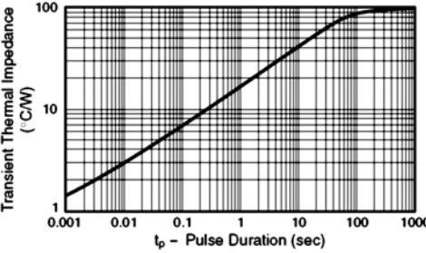
Fig. 8 – Typ. Transient Thermal Impedance
