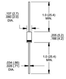
DO-204AL (DO-41)
