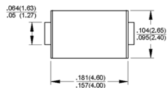
DO-214AC (SMA)
