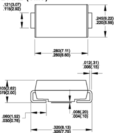
DO-214AB (SMC)
